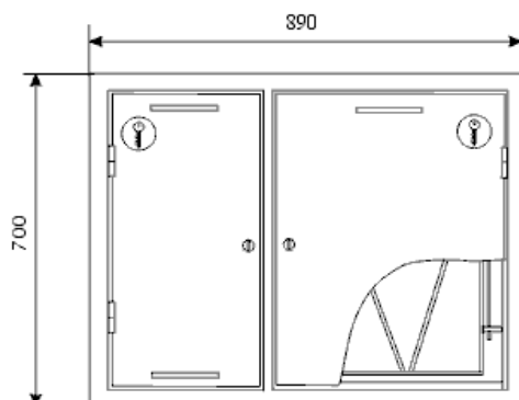
Шкаф пожарный ШП-02ВЗ (диам. 51/66 мм)
