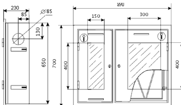
Шкаф пожарный ШП-02ВО (диам. 51/66 мм)
