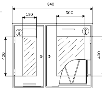
Шкаф пожарный ШП-02НО (диам. 51/66 мм)
